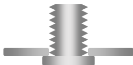
Reverse weld: Stud
